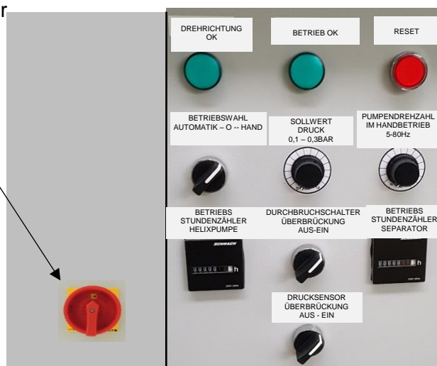
Abbildung 8 Schaltschrank
