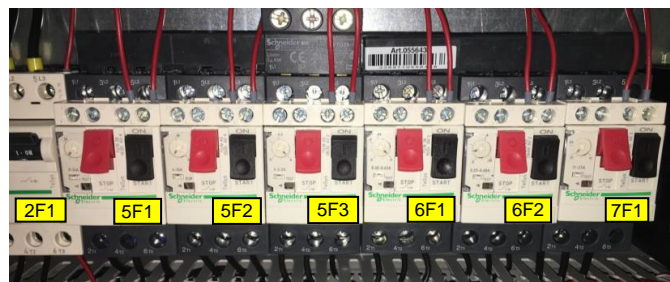
Abbildung 24 Motorschutzschalter
