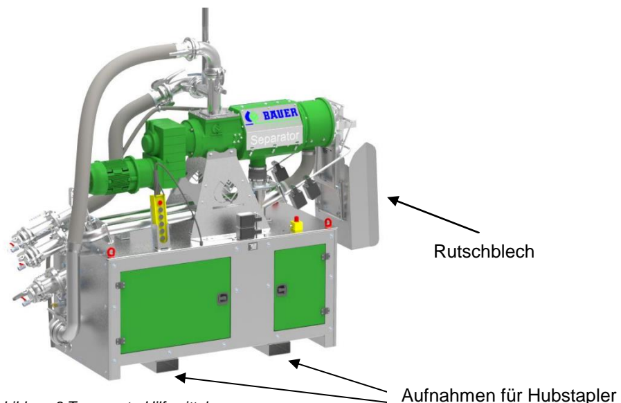
Abbildung 3 Transport - Hilfsmittel
