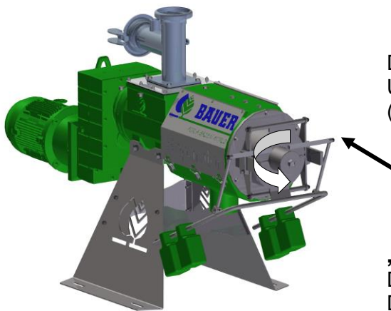
Abbildung 6 Drehrichtung Separator Schnecke
