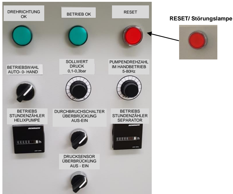
Abbildung 13 RESET Knopf Störungslampe
