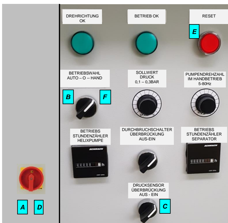
Abbildung 12 Fehlerüberbrückung Drucksensor
