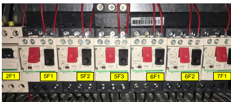
Abbildung 7 Motorschutzschalter
